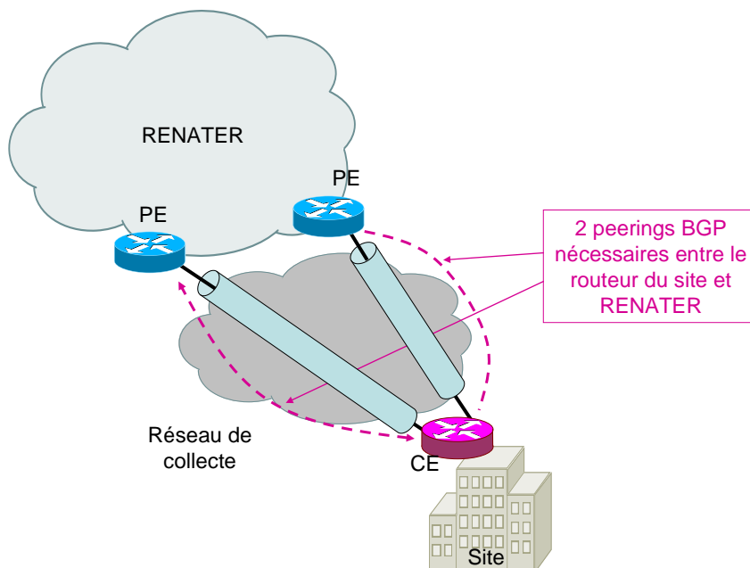
Figure 6 - Connexion redondée via la création de 2 tunnels points-à-point sur le réseau de collecte (VLANs, L2VPN MPLS...)
