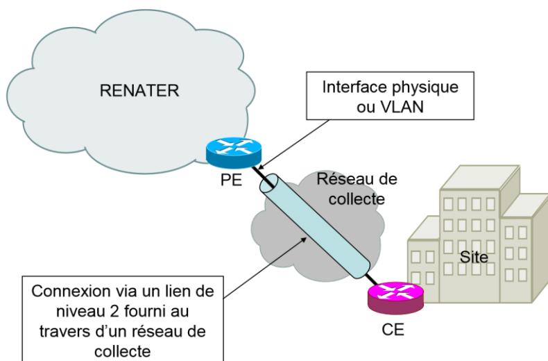
Figure 3 - Connexion via une liaison directe
